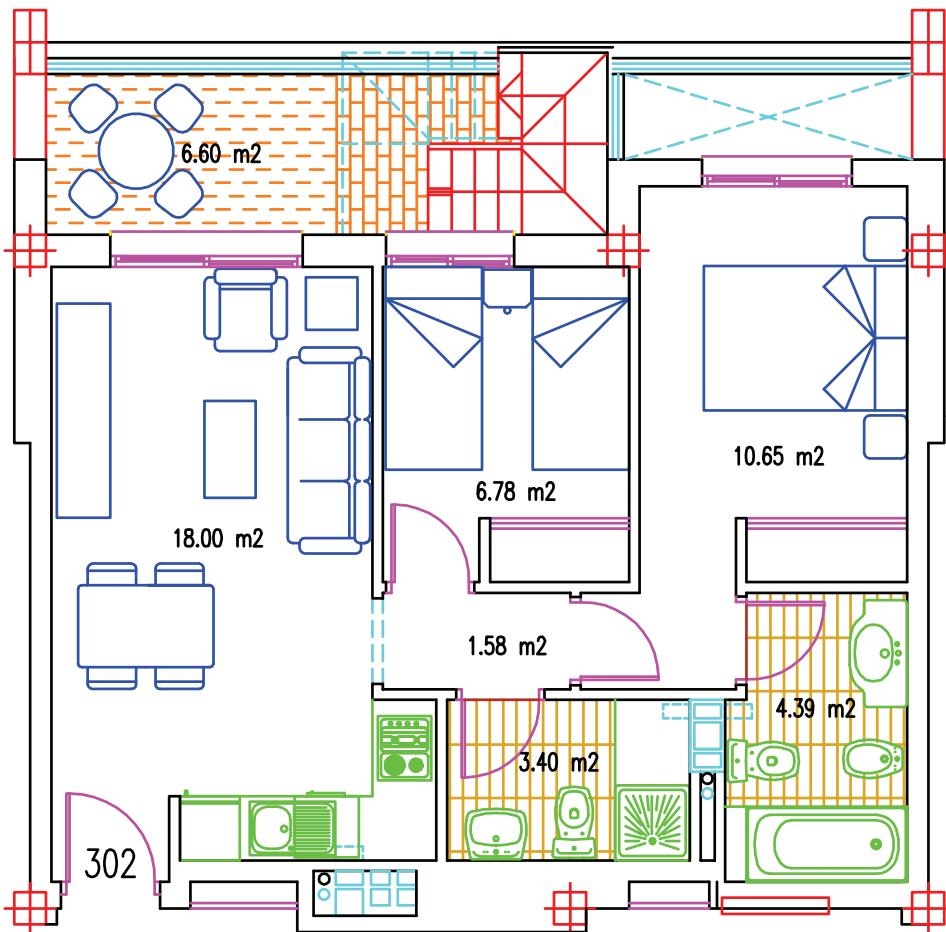
PLANTA TERCERA
