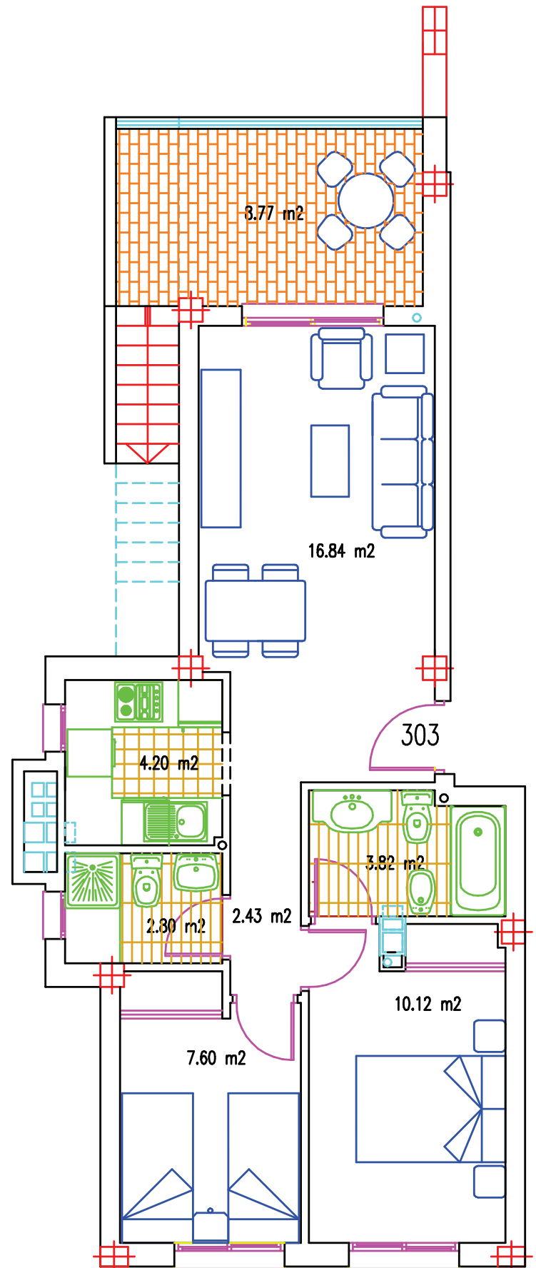
PLANTA TERCERA
